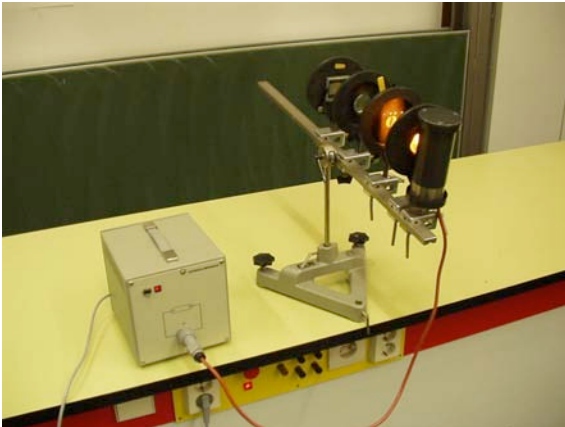
Abb. 6: Untersuchung der Spektren verschiedener Lichtquellen
