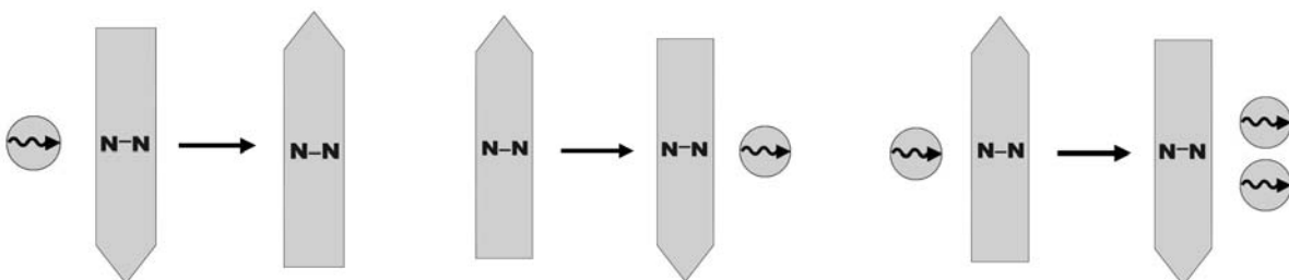
Abb. 5: Absorption, spontane Emission und stimulierte Emission im Pfeilmodell
